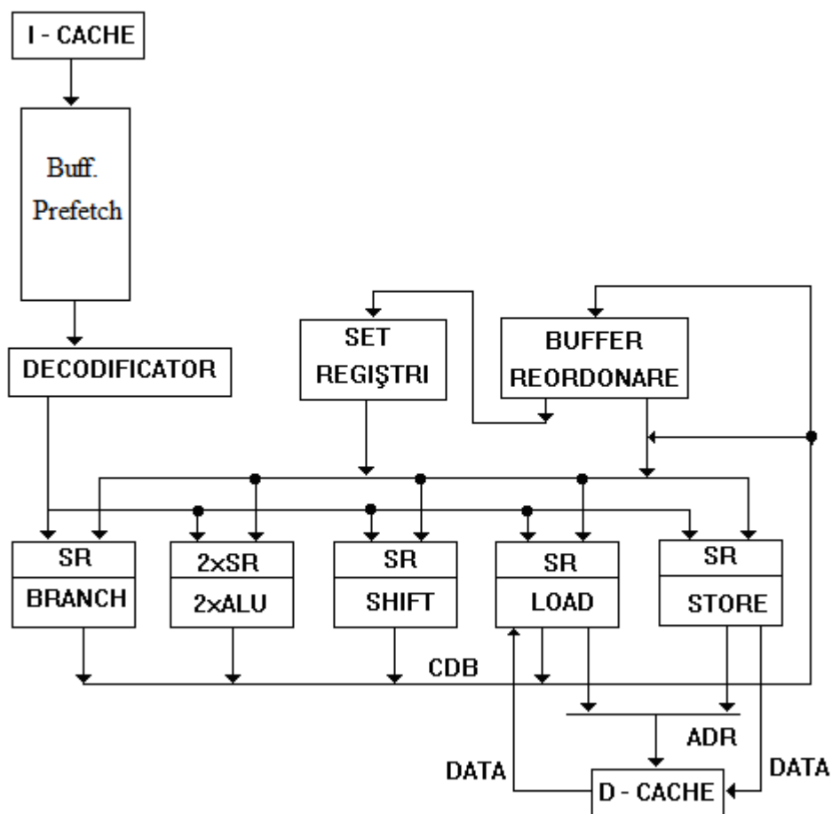
Figura 1. Schema bloc a unui microprocesor superscalar
